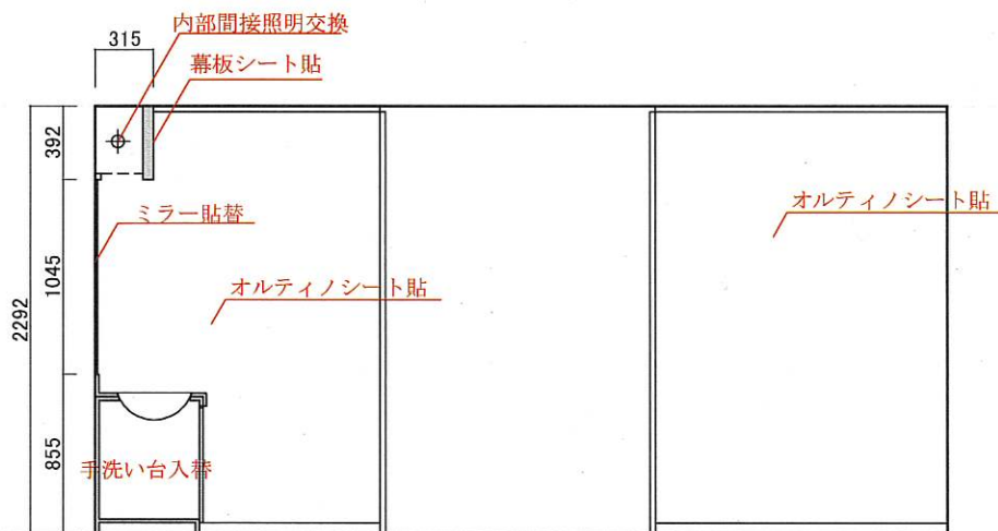
展開図B-1
