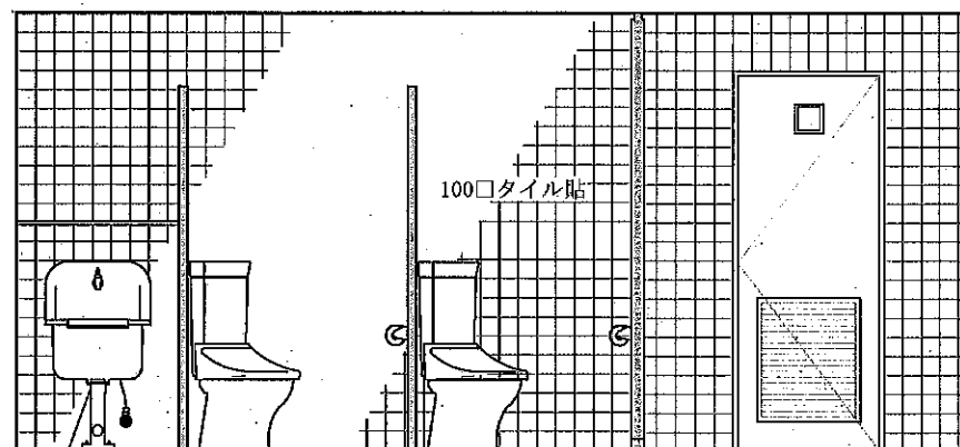
展開図C-2
