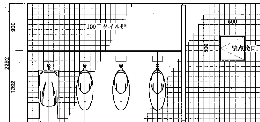
展開図C
