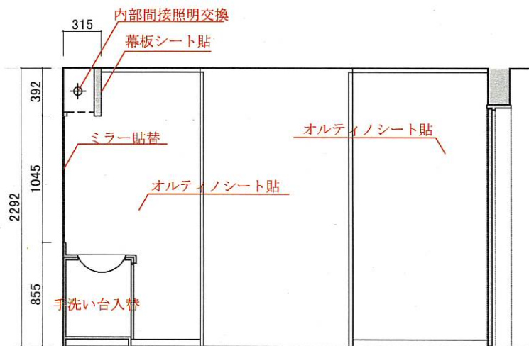
展開図B-1
