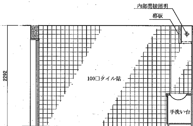
展開図D-1
