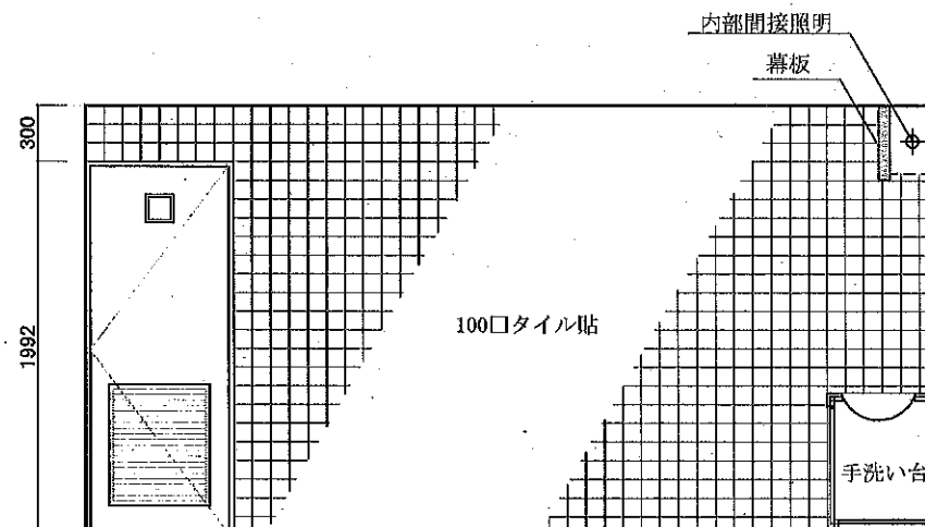
展開図D-2
