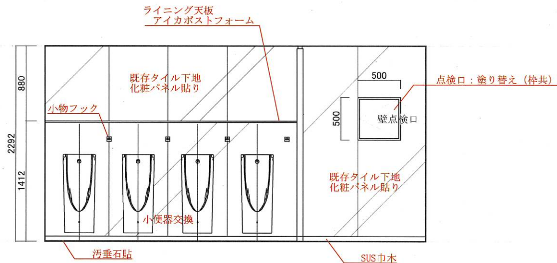
展開図C
