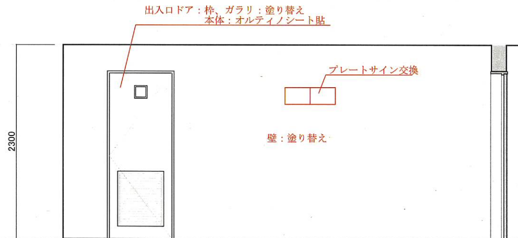
展開図A
