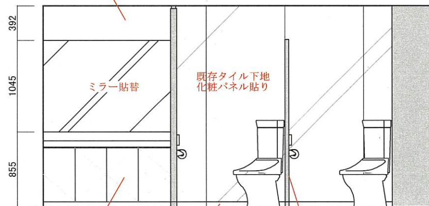
展開図A-2
