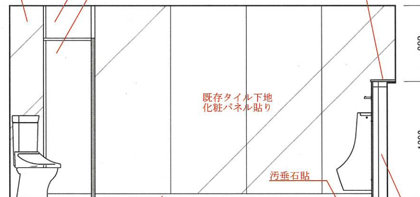
展開図B-2
