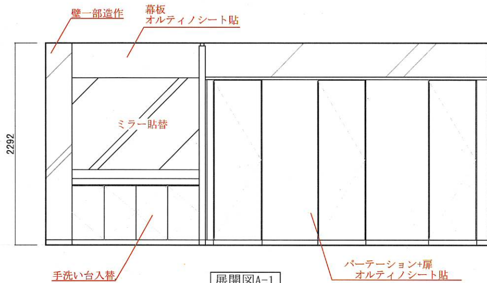
展開図A-1
