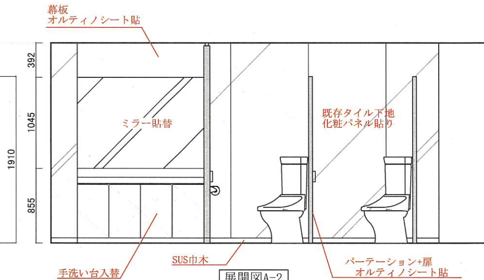
展開図A-2
